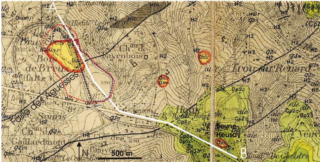
Figure 2 : Le Verger de Fayenbois dans son contexte géologique (Fond de carte extrait de la carte géologique, planchette de Seraing-Chênée ; Forir, 1897).
