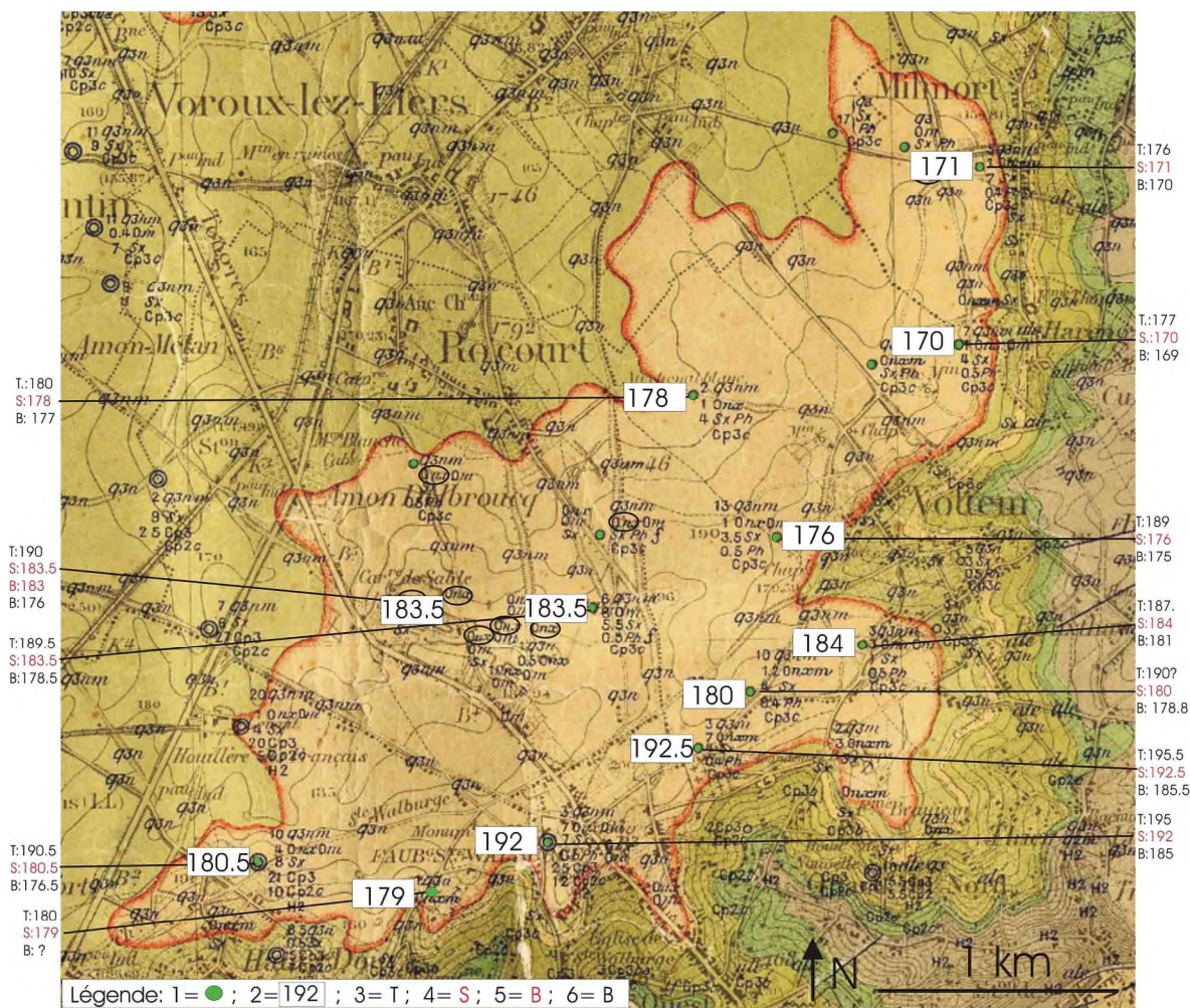
Figure 17 : Altitude en mètre du cailloutis Onx et du sable marin Om sur le plateau de Rocourt-Milmort. Légende : 1 = donnée du Service géologique de Belgique ; 2 = mise en évidence de l'altitude du toit du cailloutis Onx ; 3 = altitude de la surface topographique ; 4 = altitude du sommet du cailloutis Onx ; 5 = éventuellement altitude de la base du cailloutis Onx ; 6 = altitude de la base du sable oligocène Om . Fond de carte géologique : plage ocre avec bande rouge = sable marin oligocène et éventuellement cailloutis Onx ; plages vertes = terrains crétacés ; plage grise = terrains houillers.
